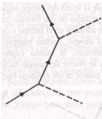
Dispersión del electrón-fotón
