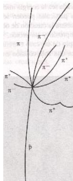
Creación de ocho piones en una colisión entre un antiprotón ( \bar{p} ) y p protón (que esperaba en la cámara de burbujas)
