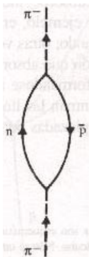
Creación de un par virtual neutrón-antiprotón
